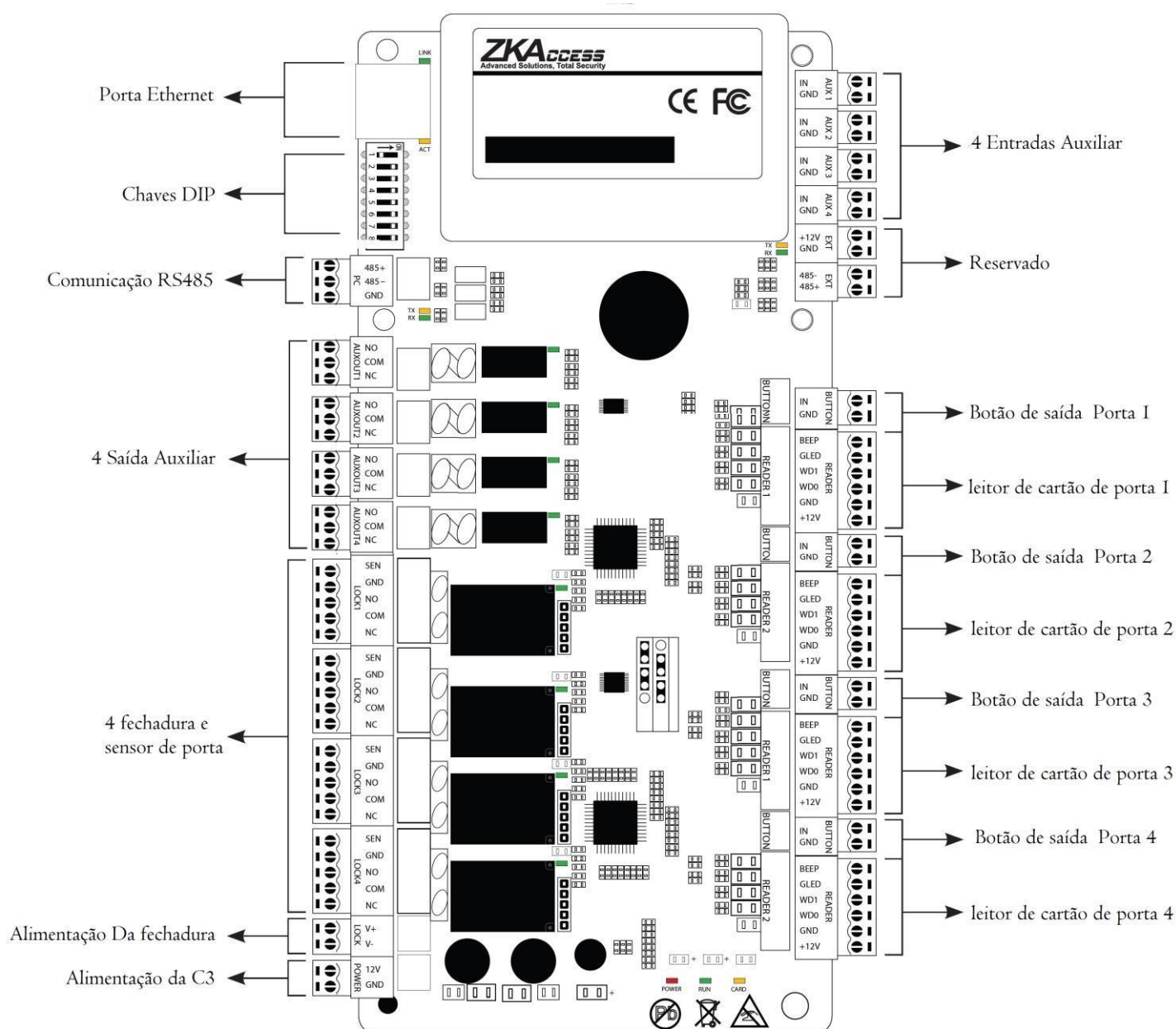
460: Diagrama dos terminais de conexão:
